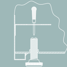
REGULAÇÃO DOS NIVELADORES PELO INTERIOR REGULACIÓN DE LOS NIVELADORES POR EL INTERIOR
